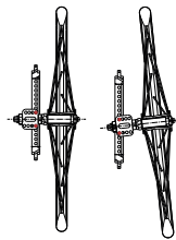
Carrossage ajustable sur le fauteuil de 0° à 6°
